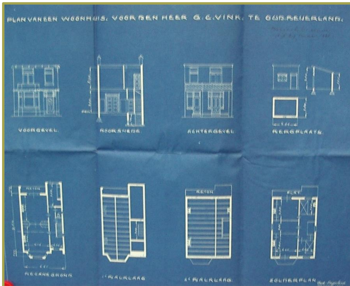
Tekening behorend bij de Bouwaanvraag van 11 februari 1927
