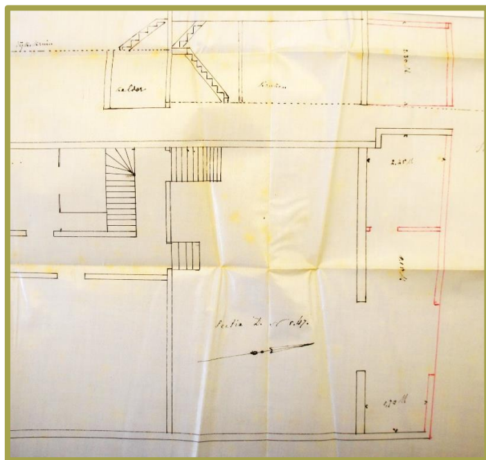
De tekening behorend bij de bouwaanvraag bij de polder Oud-Beijerland. Rechts op de tekening de uitbreiding.
