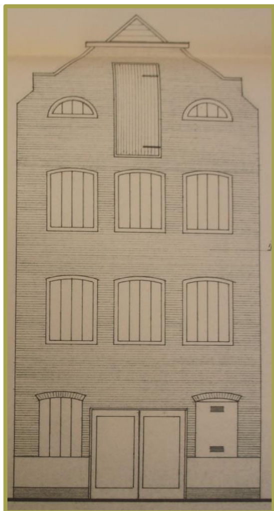
Bestaande situatie Bierkade
